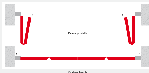
Planta (instalação dentro vão na largura)
